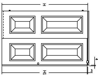
DIMENSIONI PANNELLO - ROZMĚRY PANELU - ROZMERY PANELU - TÜRMASSE - DOOR DIMENSIONS
